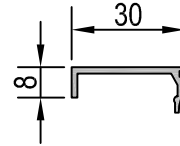
Bauanschlußprofil bei WL 65/75
